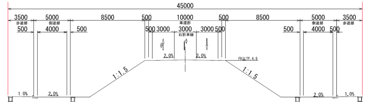
高盛土交差点部 (K-K断面)
