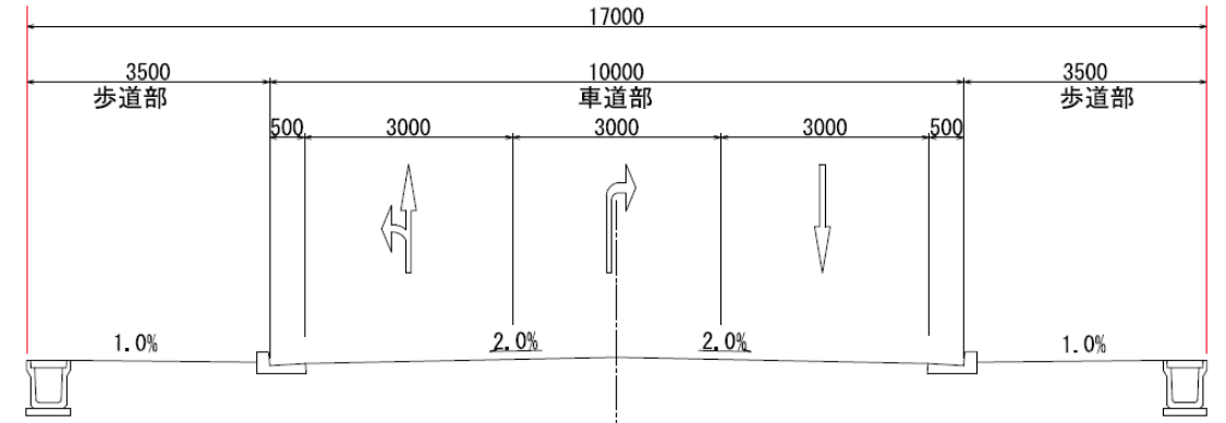
高盛土部 (J-J断面)
