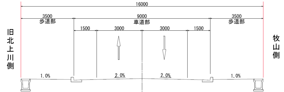
交差点部 (I-I断面)
