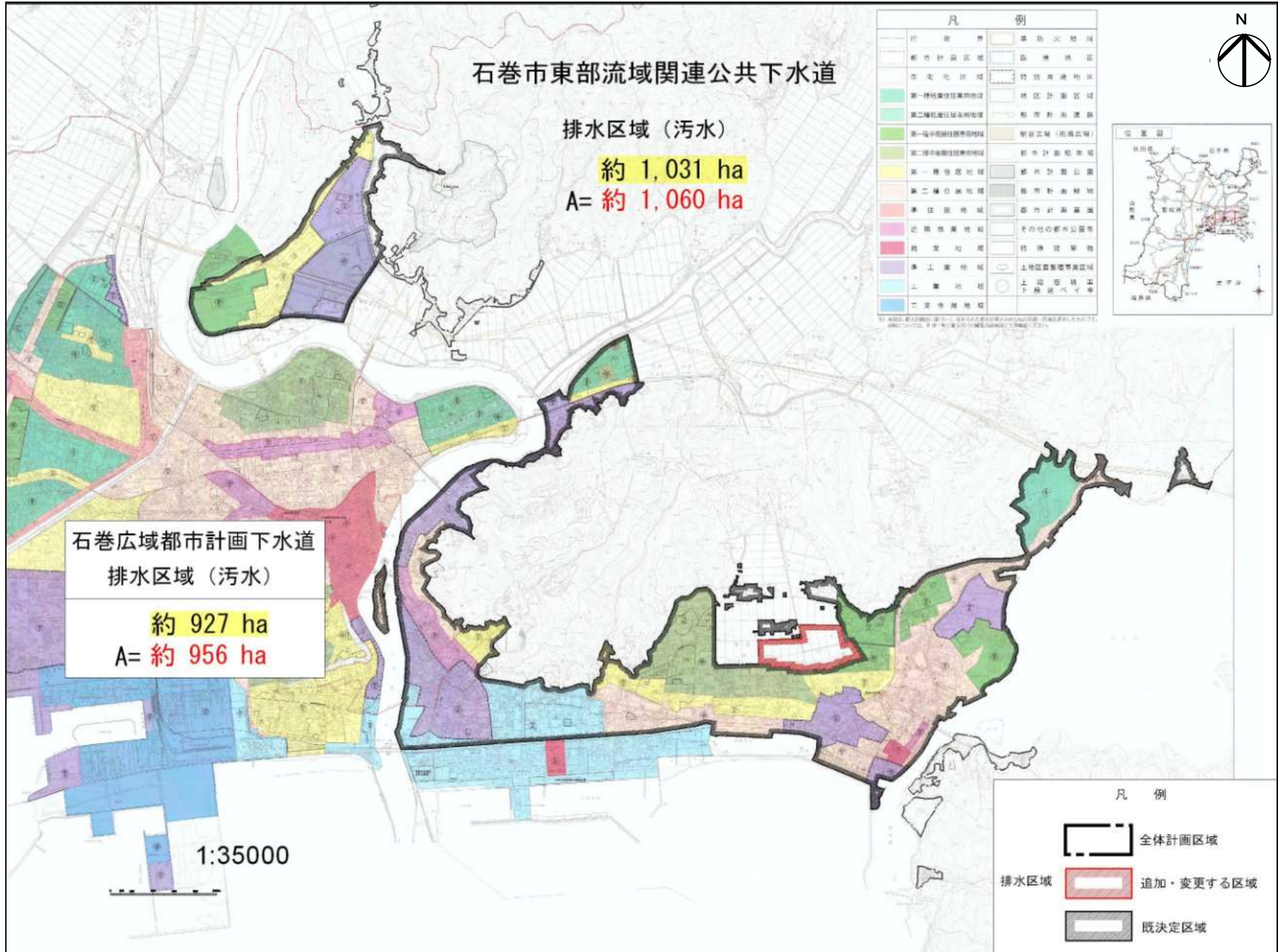
石巻広域都市計画及び河北都市計画下水道の変更（石巻市決定） （石巻市東部流域関連公共下水道の変更） 総括図
