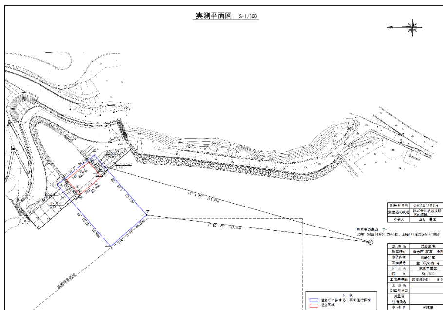
実測平面図
