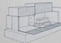
横口式石標
