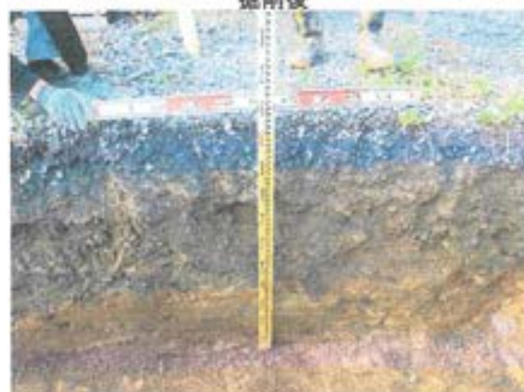
断面
