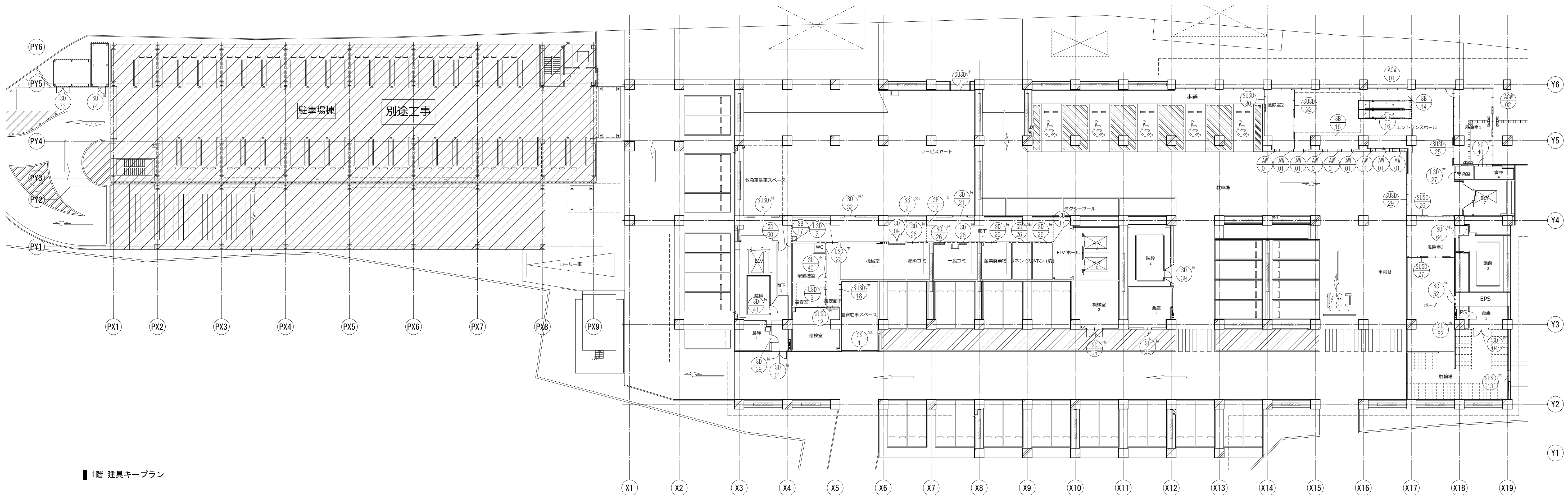
2階 建具キープラン
