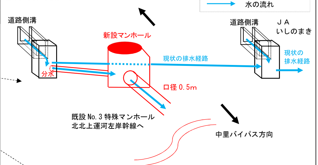
接続箇所イメージ図
