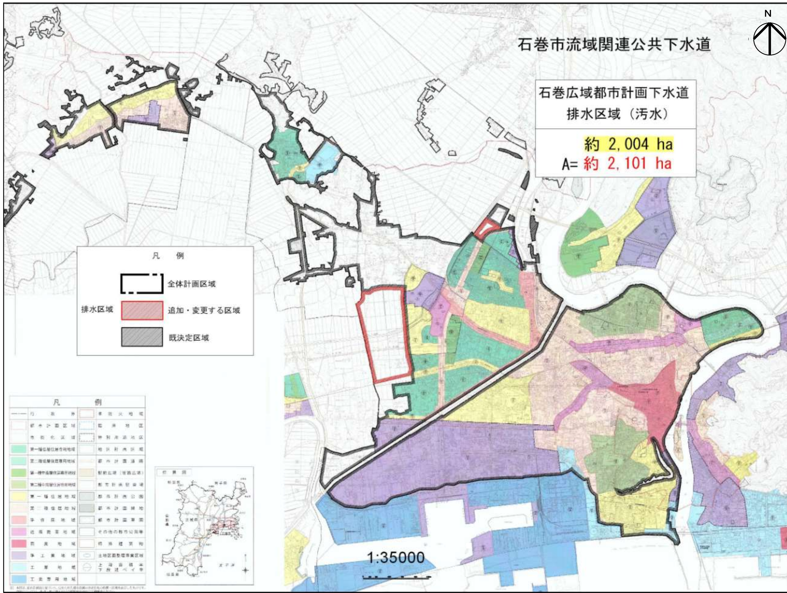
石巻広域都市計画下水道の変更 (石巻市決定) (石巻市流域関連公共下水道の変更) 総括図
