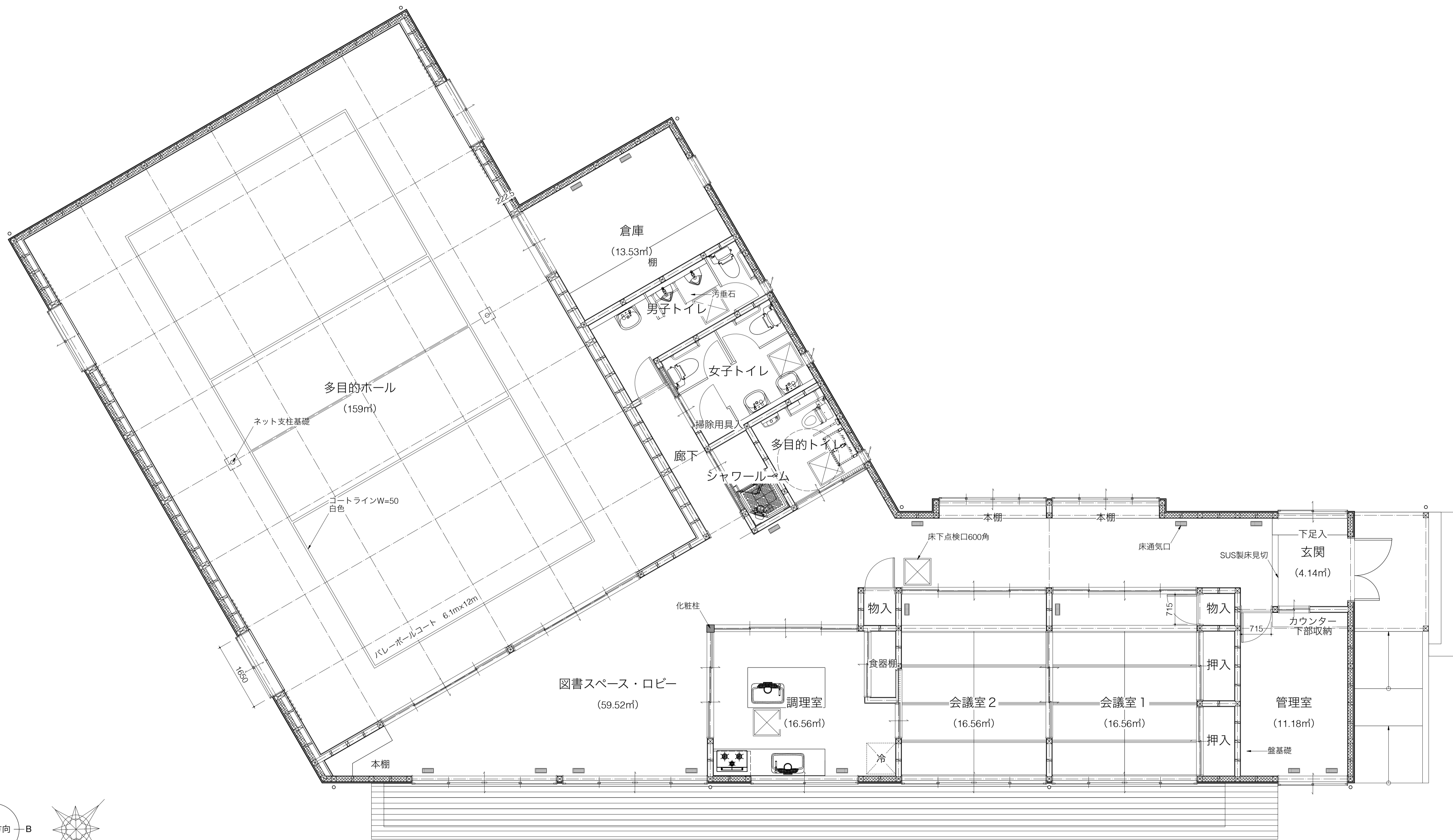
1 平面詳細図 - 1:50
