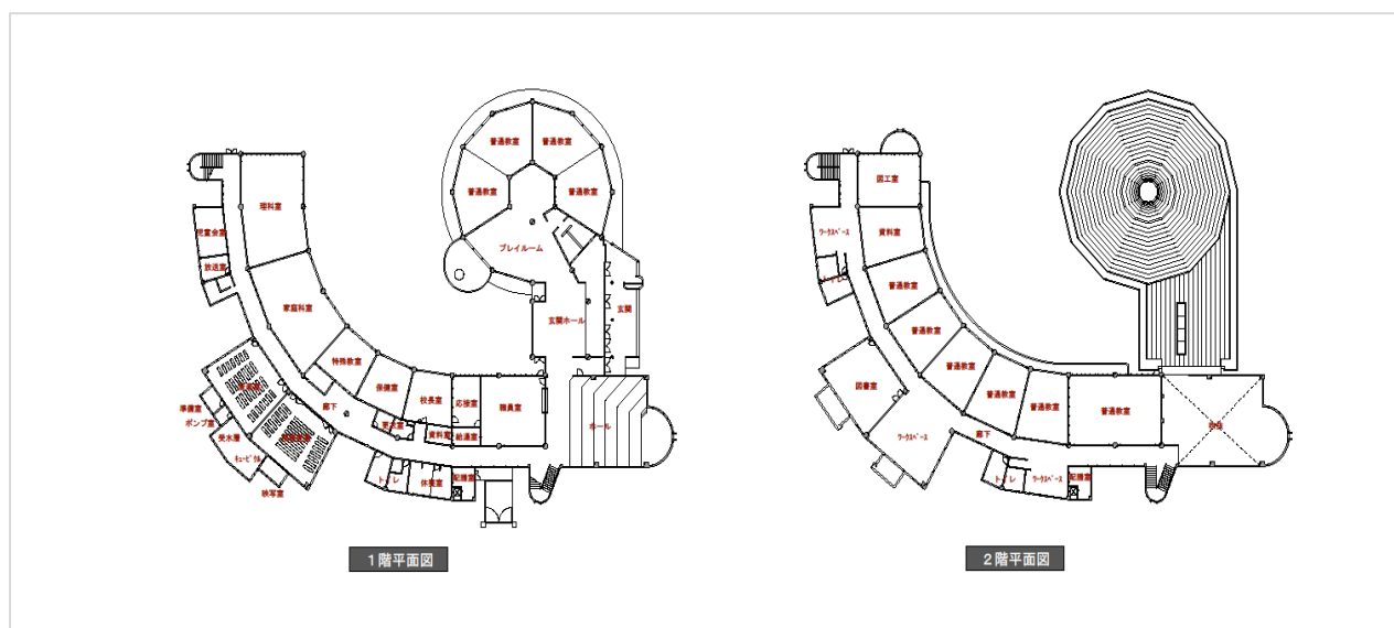
<校舎平面図>
