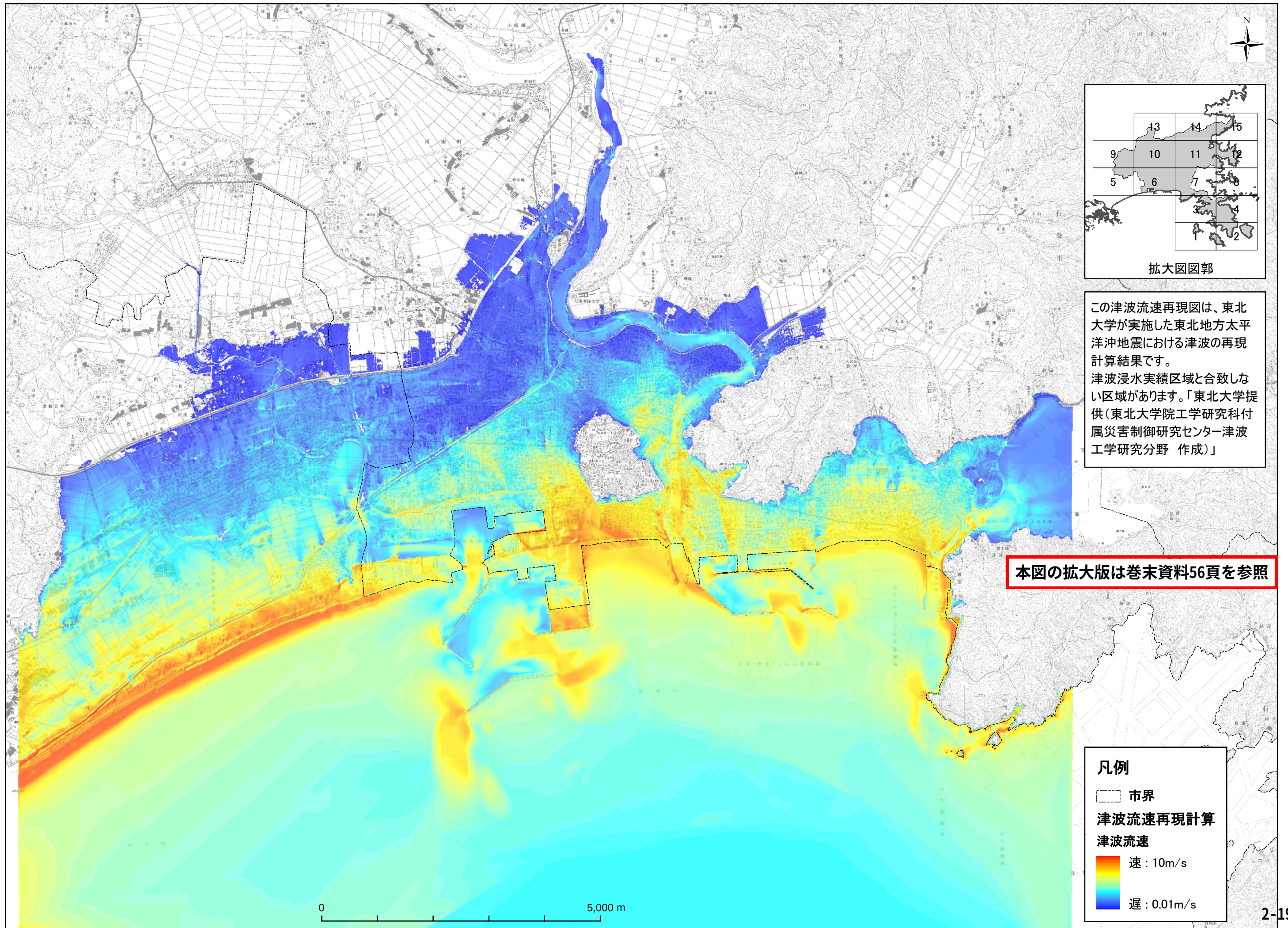
図2-14 津波流速再現計算
