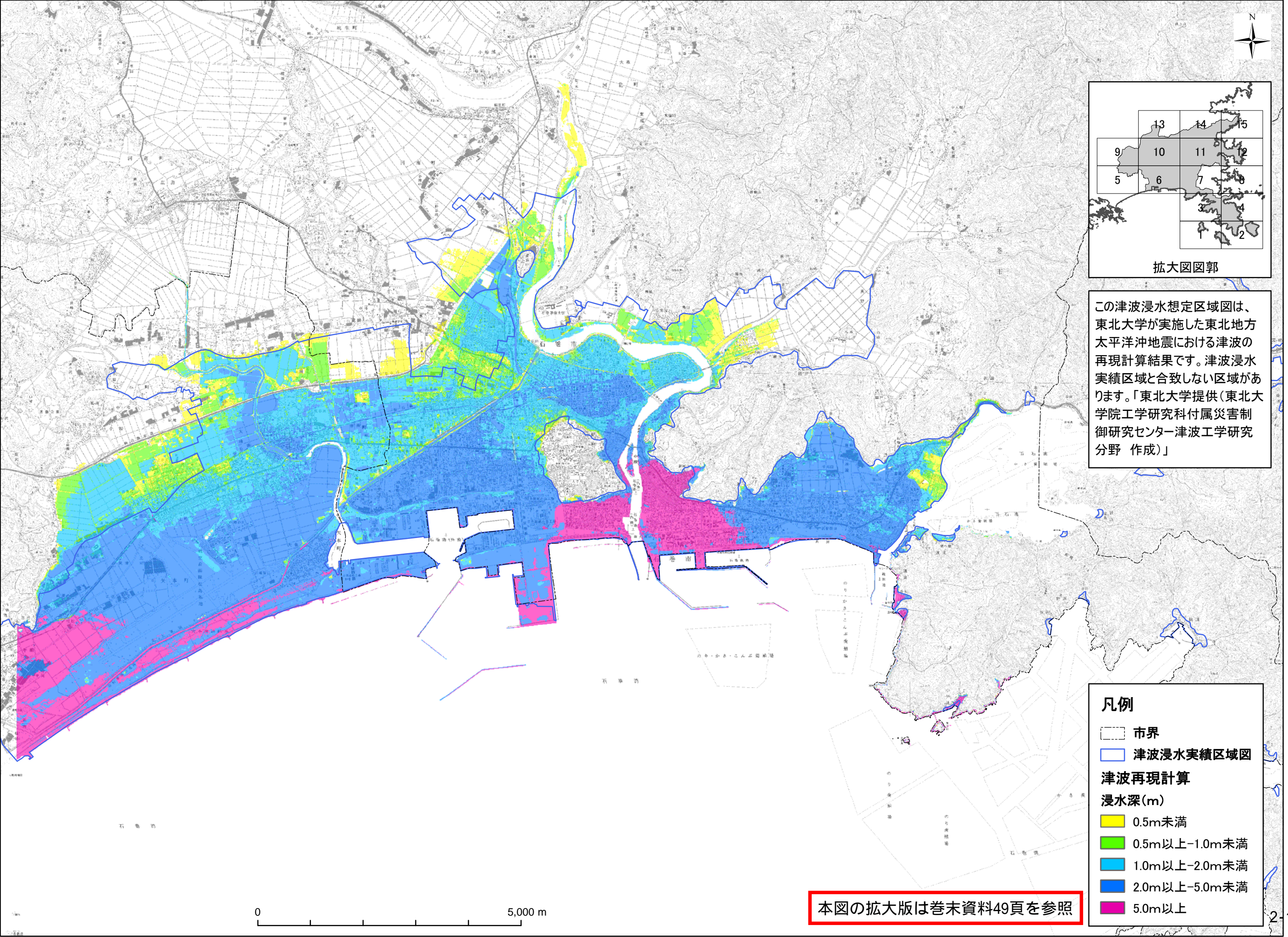
図2-13 津波再現計算
