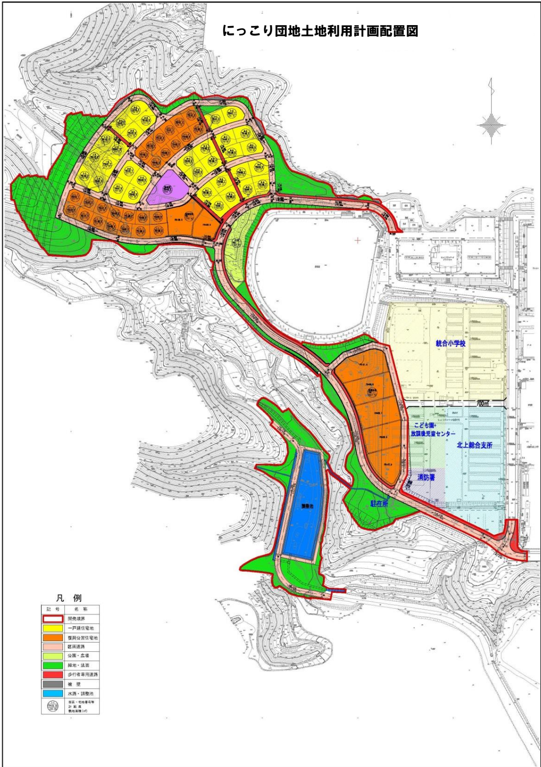
土地利用計画平面図
